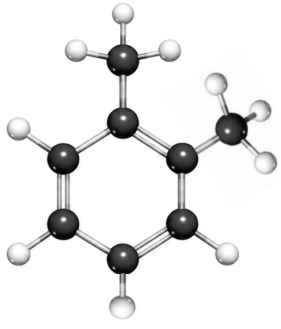
অর্থো- জাইলিন
