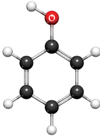
ফেনল
