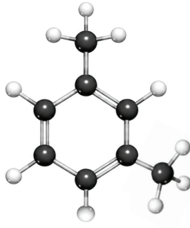
মেটা- জাইলিন
