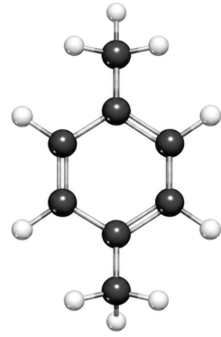
প্যারা- জাইলিন
