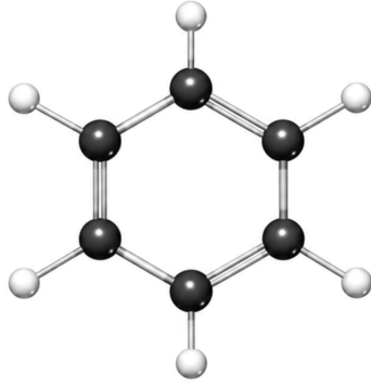
বেনজিন
