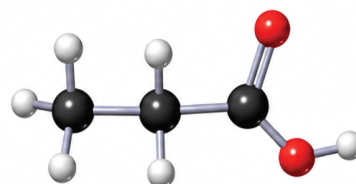
প্রোপানোয়িক এসিড
