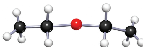
ডাইইথাইল ইথার
