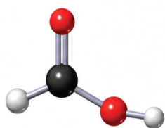
মিথানোয়িক এসিড
