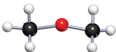
ডাইমিথাইল ইথার
