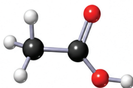
ইথানোয়িক এসিড
