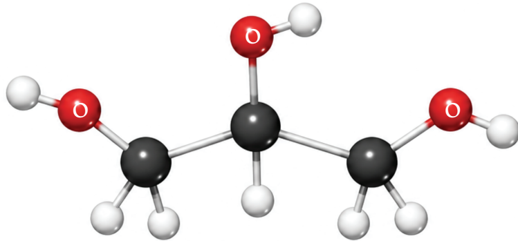
গ্লিসারিন (গ্লিসারল)
