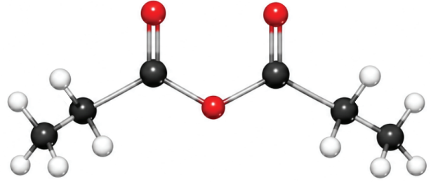
প্রোপানোইক অ্যানহাইড্রাইড
