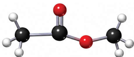
মিথাইল অ্যাসিটেট
