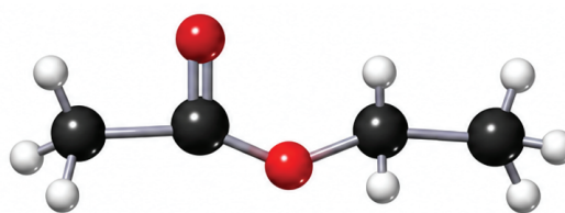
ইথাইল অ্যাসিটেট
